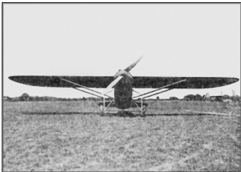
Avion Latécoère 28 (1 moteurs 500 CV) (de la Compagnie Générale Aéropostale. Lignes d'Afrique) (Cet avion est l'avion commercial le plus rapide du monde)
